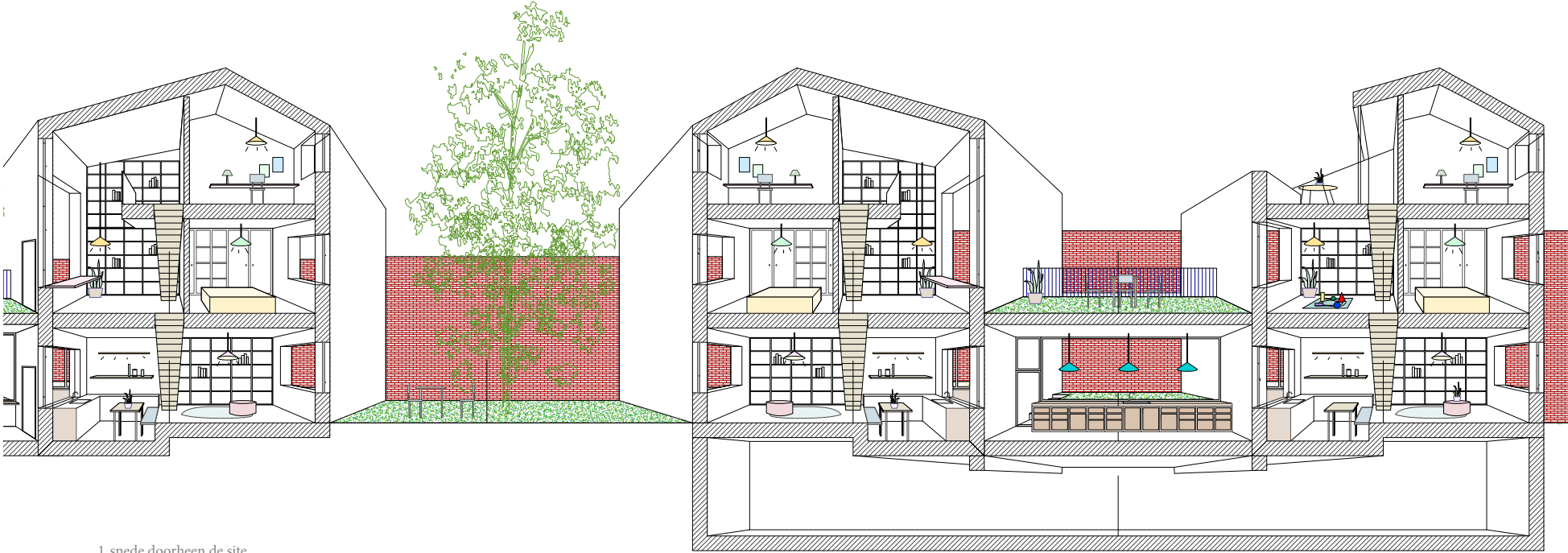
1 snede doorheen de site
